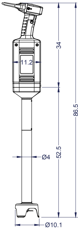
Vista Elevación
