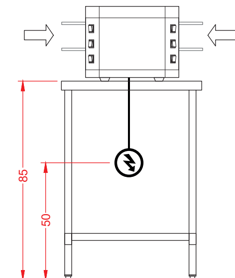
Vista Izquierda
