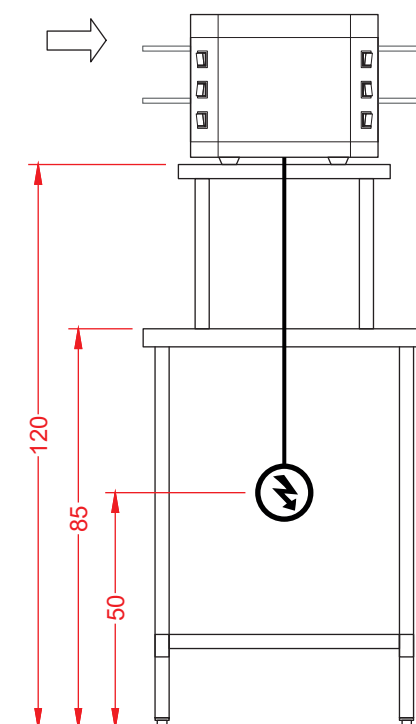
Vista Izquierda
