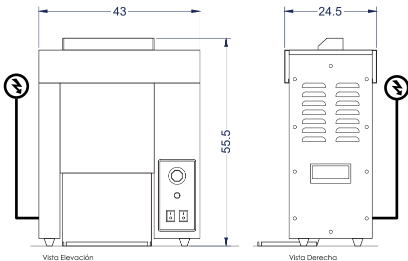
Vista Elevación
