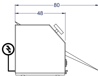
Vista Izquierda
