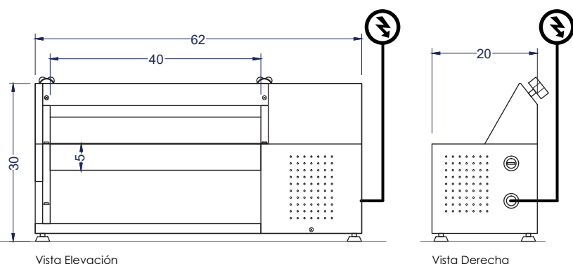
Vista Elevación
