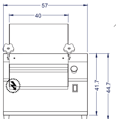
Vista Elevación
