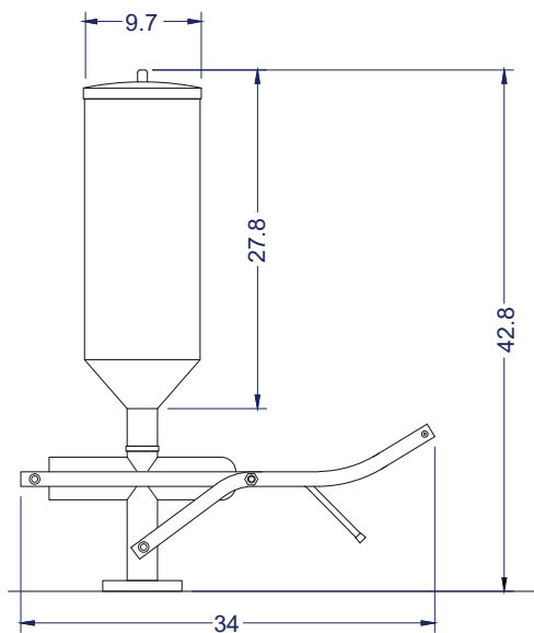
Vista Izquierda
