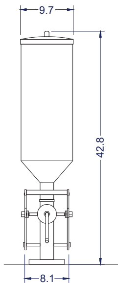
Vista Elevación
