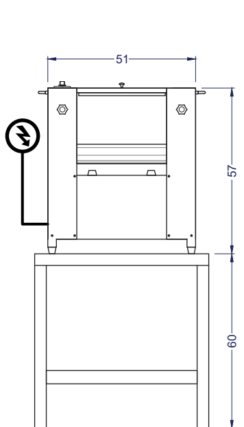
Vista Elevación
