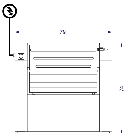
Vista Elevación
