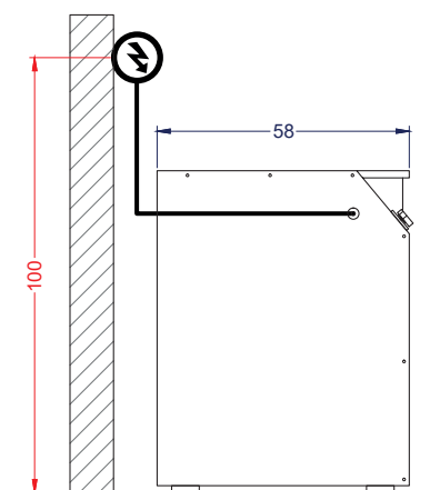
Vista Izquierda
