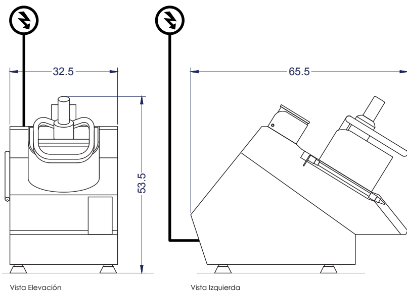
Vista Elevación
