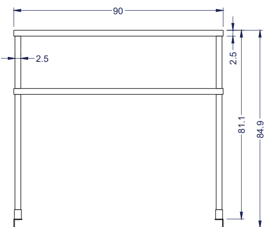
Vista Elevación
