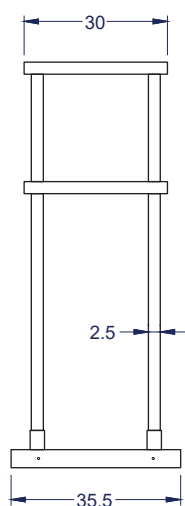
Vista Izquierda
