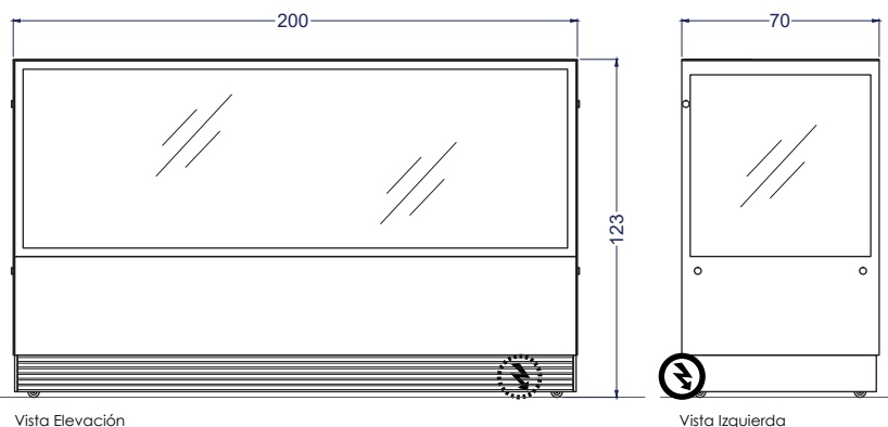
Vista Elevación
