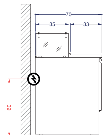
Vista Izquierda
