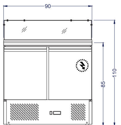
Vista Elevación
