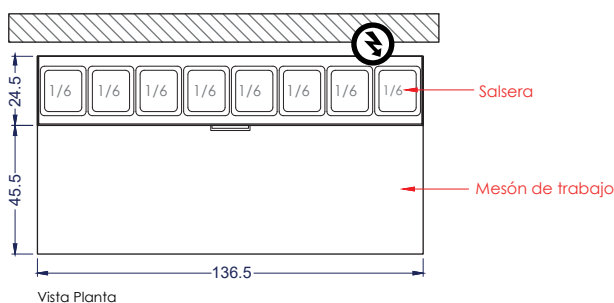
Vista Planta
