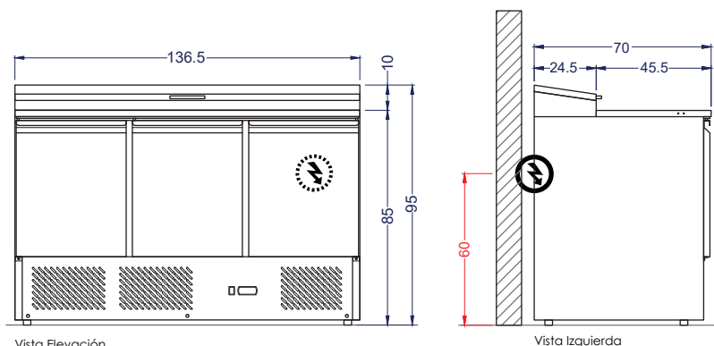
Vista Elevación
