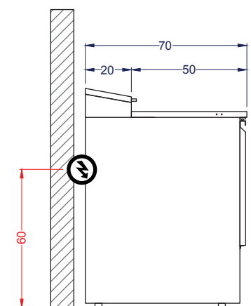
Vista Izquierda
