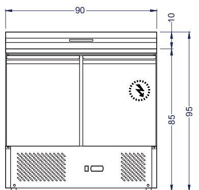
Vista Elevación
