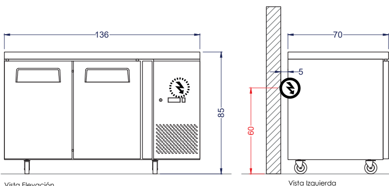
Vista Elevación
