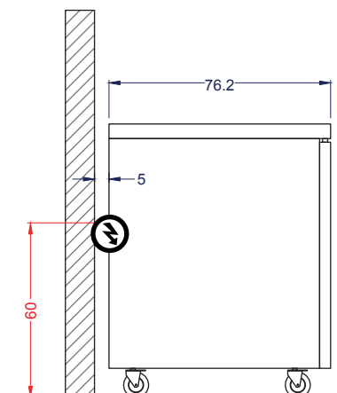
Vista Izquierda
