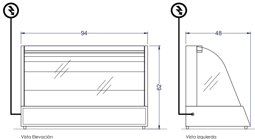
Vista Elevación
