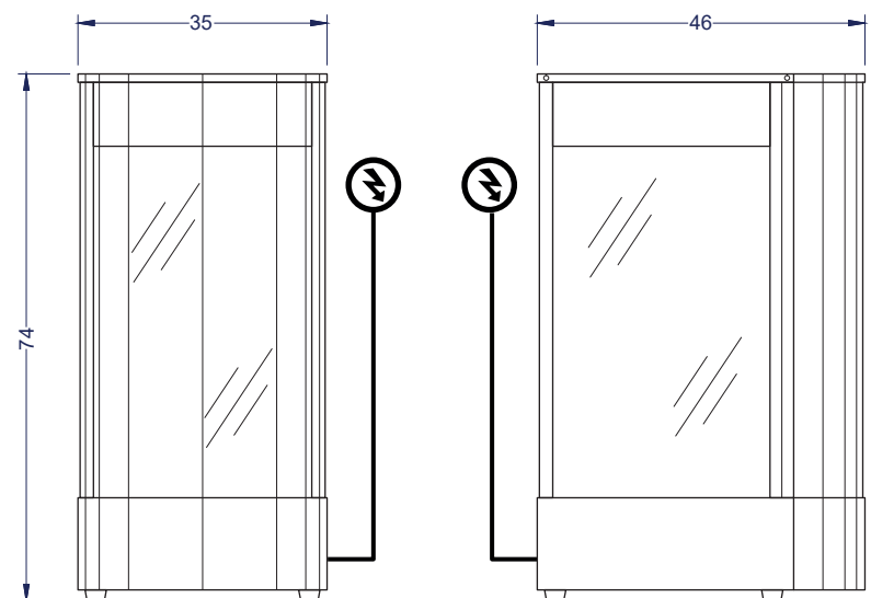
Vista Elevación
