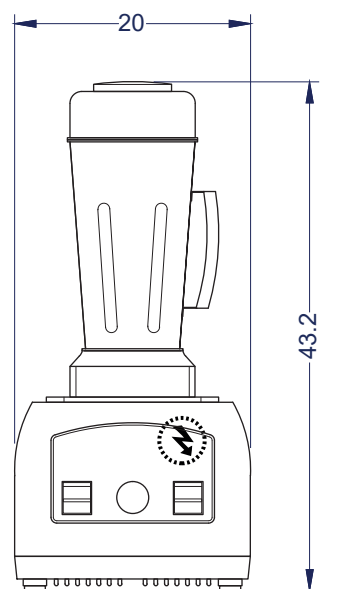
Vista Elevación
