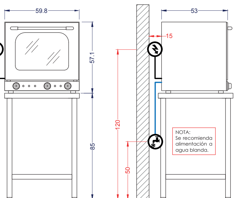
Vista Elevación
