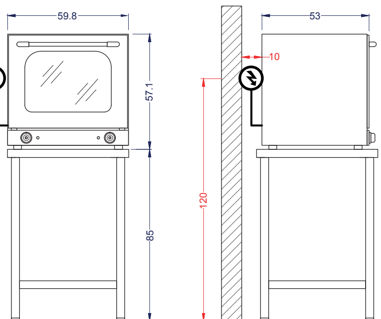
Vista Elevación
