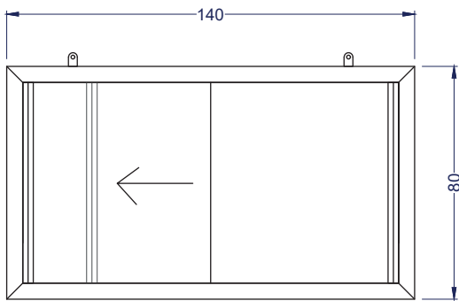
Vista Elevación
