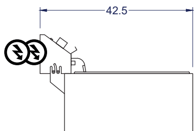
Vista Izquierda
