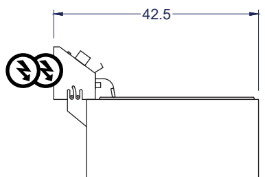
Vista Izquierda
