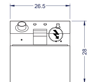
Vista Elevación
