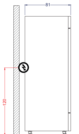
Vista Izquierda
