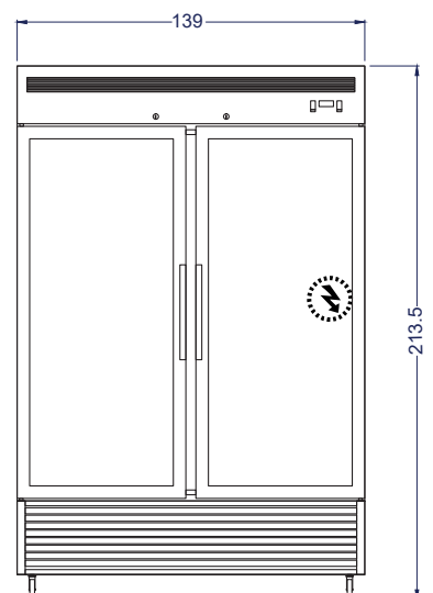
Vista Elevación
