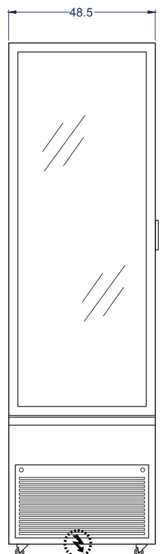
Vista Izquierda
