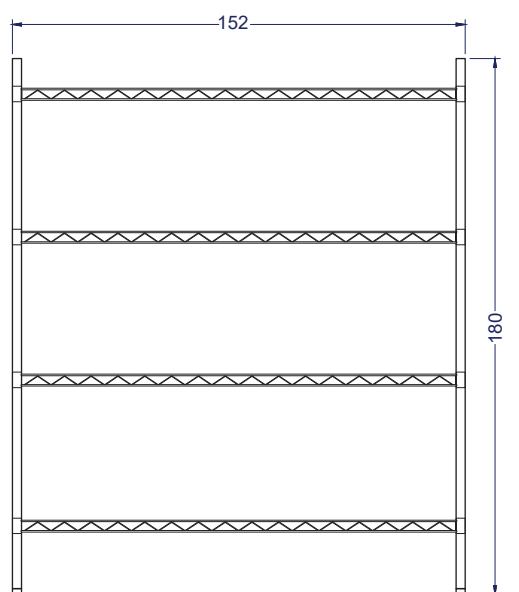
Vista Elevación
