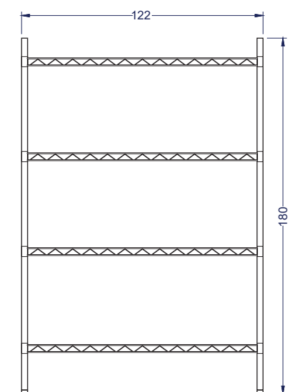
Vista Elevación
