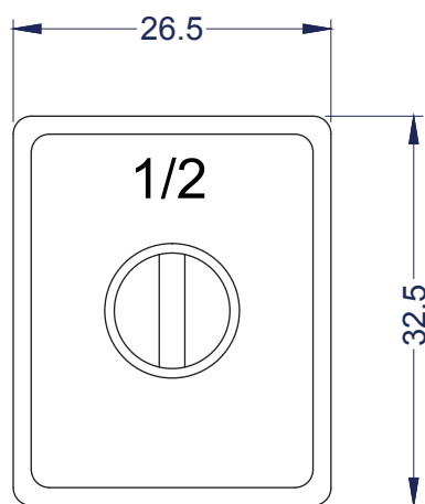
Vista Planta
