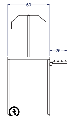
Vista Izquierda
