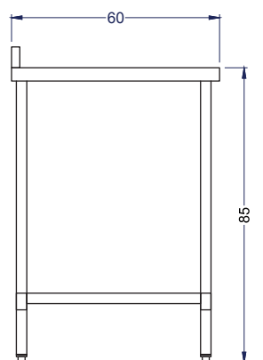
Vista Izquierda
