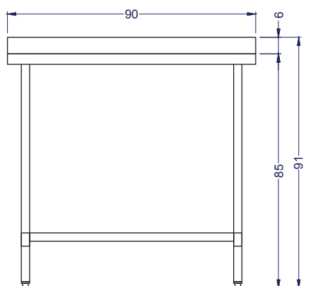
Vista Elevación
