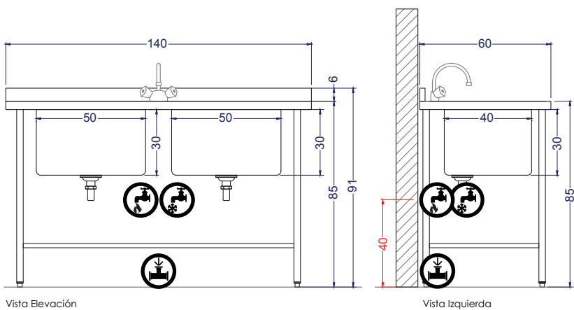
Vista Elevación
