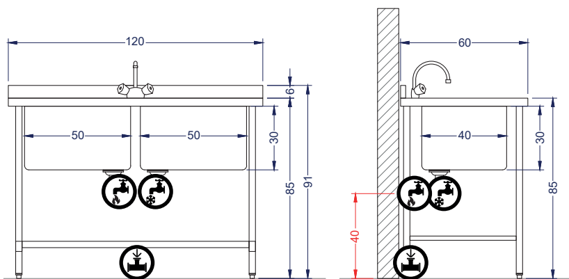
Vista Elevación
