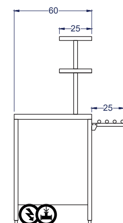
Vista Izquierda
