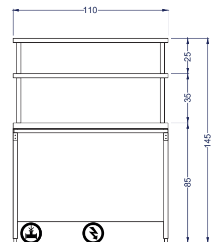
Vista Elevación
