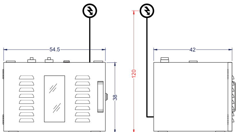
Vista Elevación
