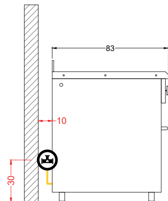
Vista Izquierda
