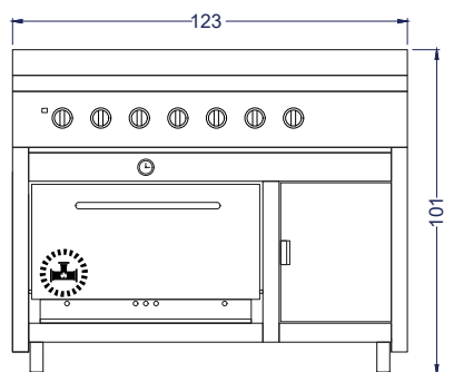
Vista Elevación
