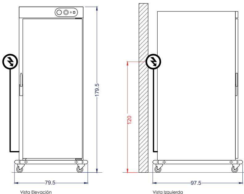
Vista Elevación
