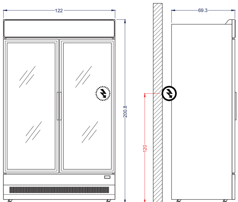
Vista Elevación
