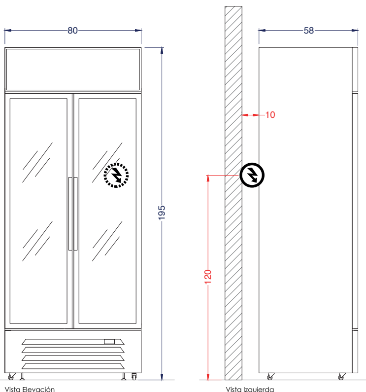
Vista Elevación
