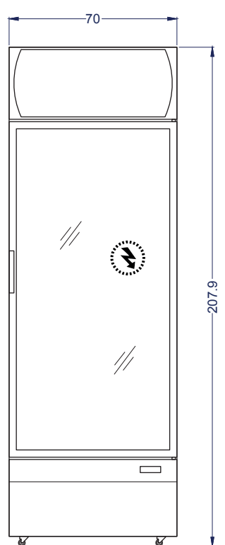
Vista Elevación
