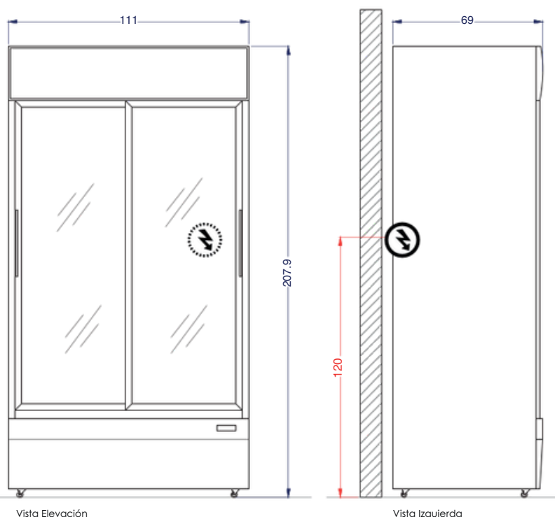
Vista Elevación
