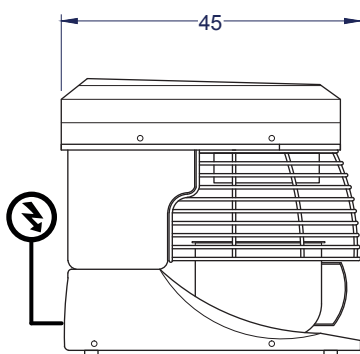
Vista Izquierda
