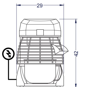
Vista Elevación
