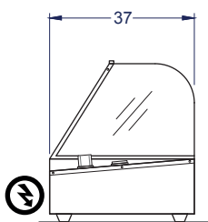
Vista Izquierda
