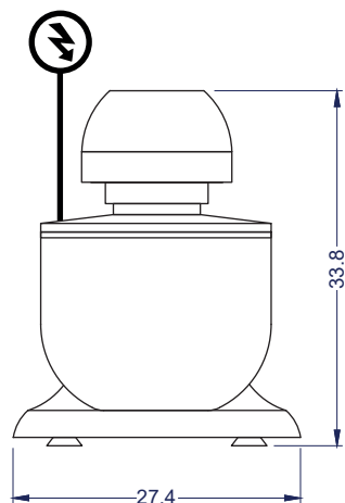
Vista Elevación
