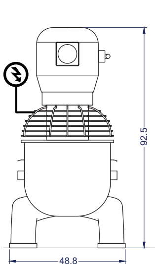
Vista Elevación
