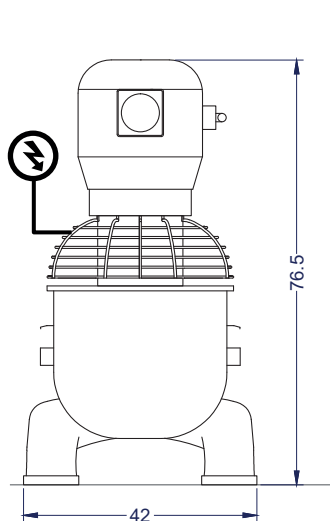
Vista Elevación
