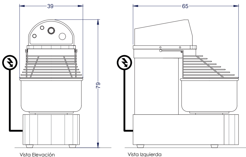
Vista Elevación
